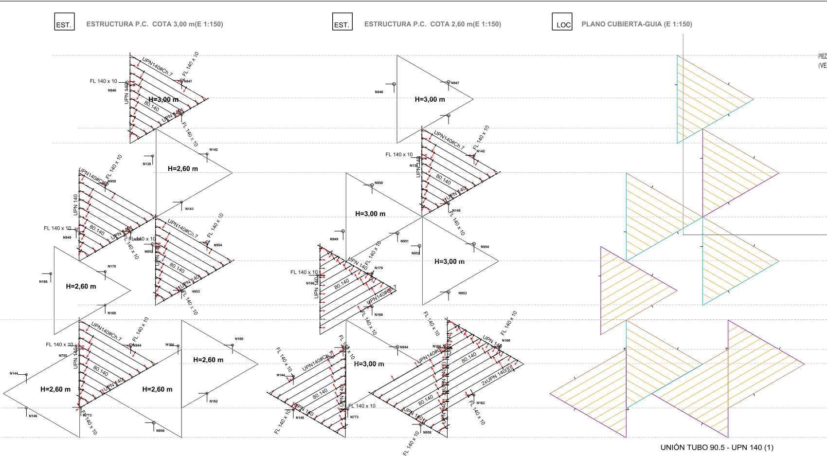
UNIÓN TUBO 90.5 - UPN 140 (1)
