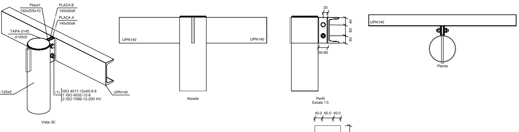
UNIÓN TUBO 125.5 - UPN 140 (1)
