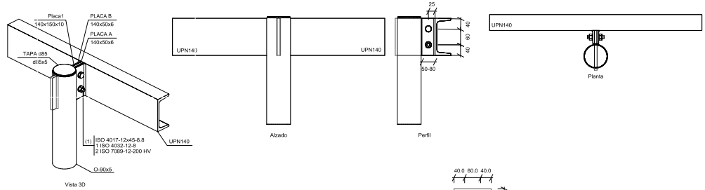
UNIÓN TUBO 90.5 - UPN 140 (1)
